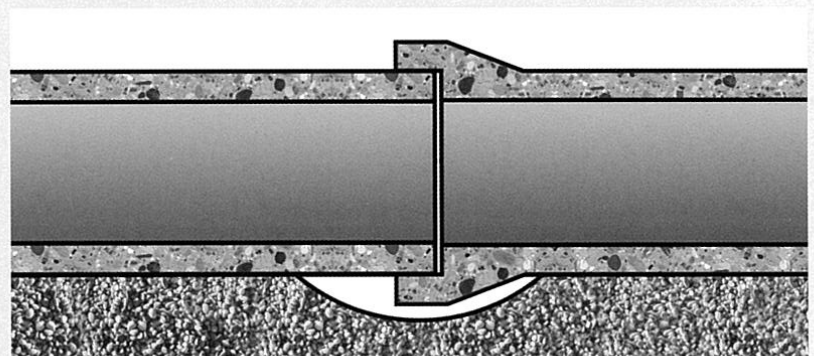
Herkömmliches Auflager
